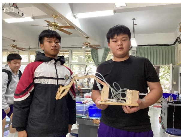
說明：液壓機械手臂設計與製作完成作品
