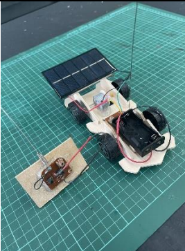
太陽能遙控汽車製作-成品展示
