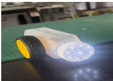
手搖發電機製作-成品展示
