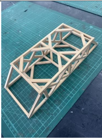
桁架橋製作-成品展示
